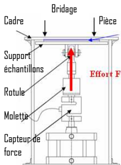
Schéma de principe de l'outillage de soudage
